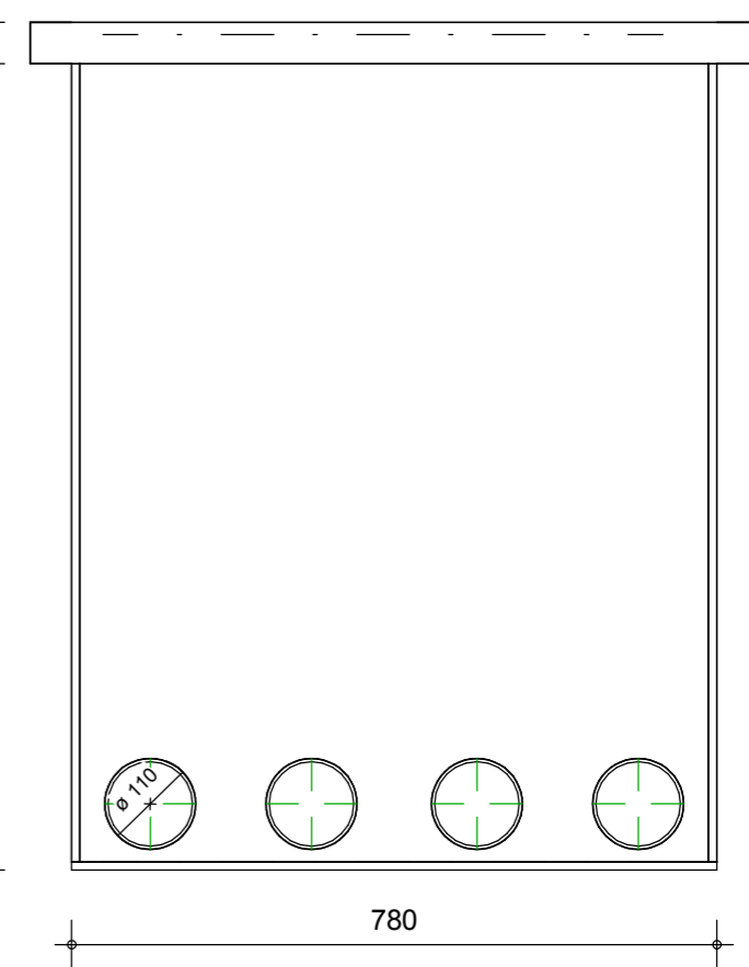
Achteraanzicht
