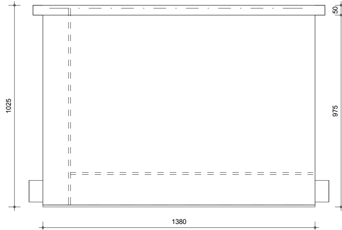
Rechter zijaanzicht
