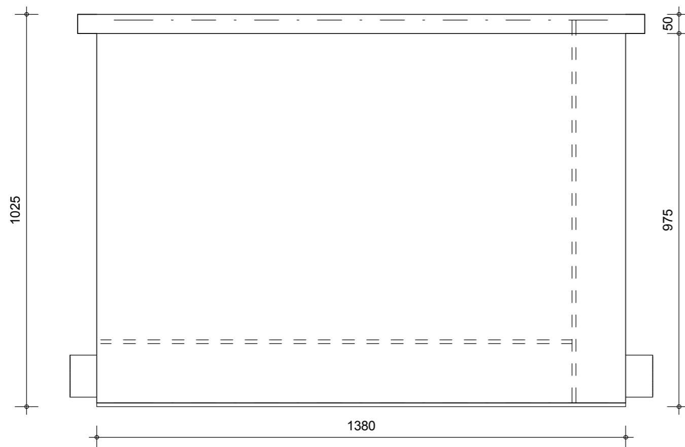
Linker zijaanzicht
