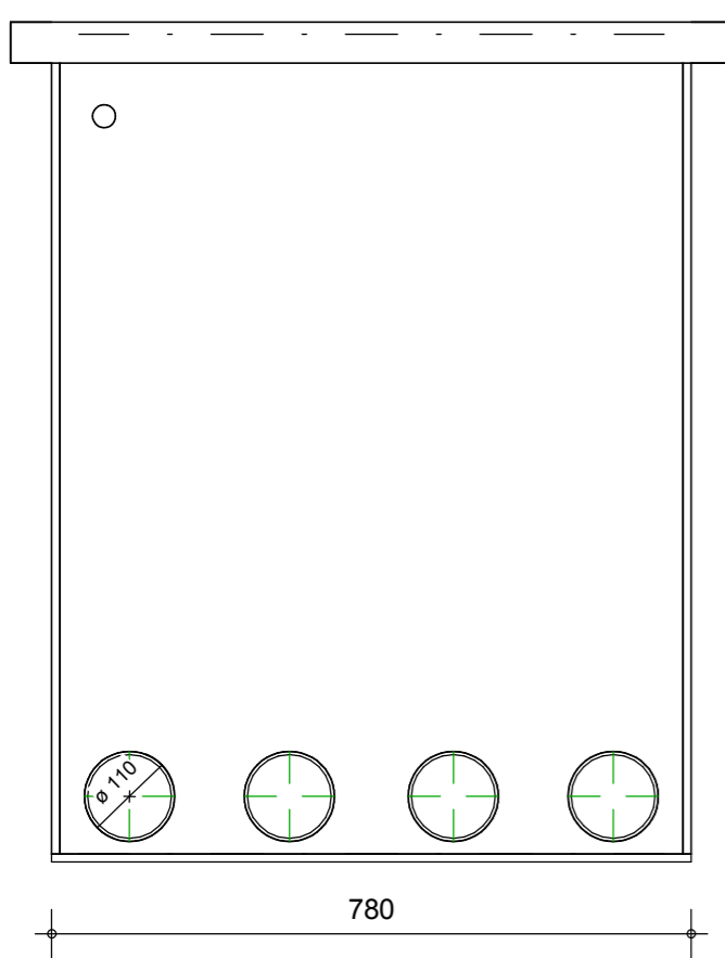
Vooraanzicht
